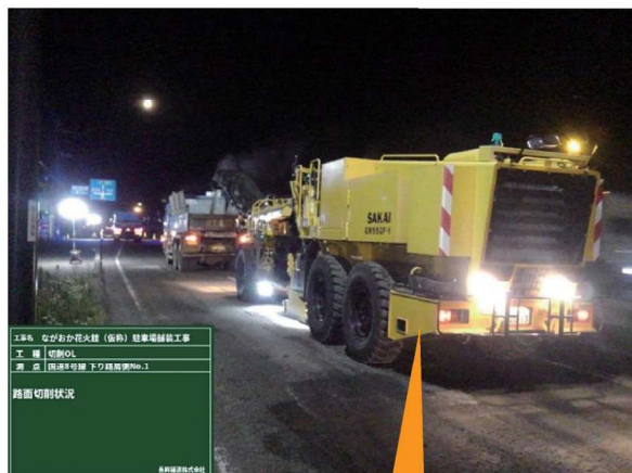
路面切削機にて 傷んだ舗装部分5cmを取除きます
